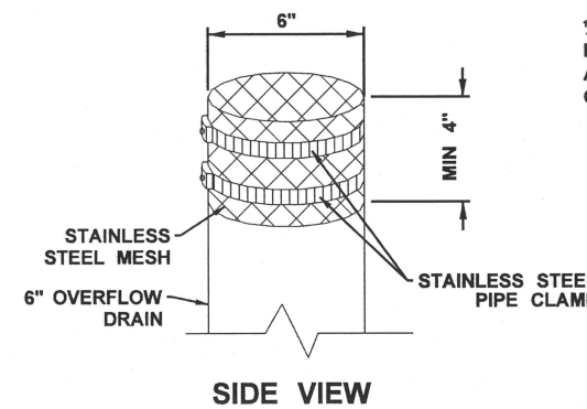
OVERFLOW DRAIN N.T.S.
