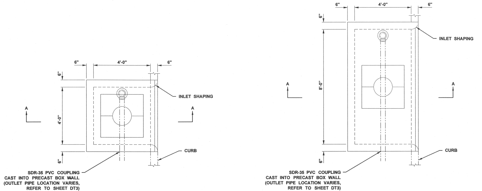
PLAN VIEW - 4'x4' FILTERRA N.T.S.
